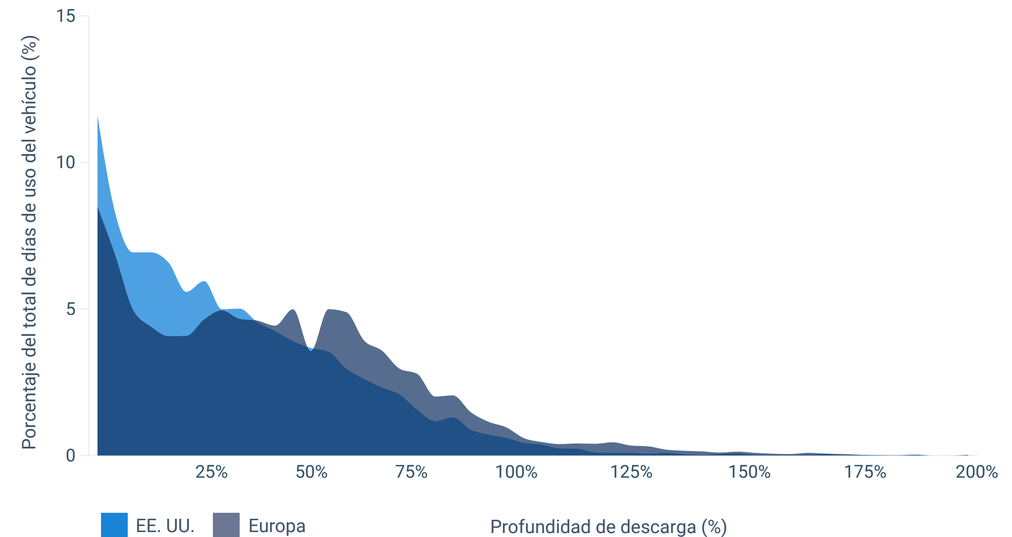
Distribución de la profundidad de descarga diaria de los vehículos eléctricos en 2025
